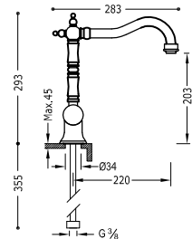
Grifo monomando para cocina Con latiguillos de alimentación flexibles G3/8.
