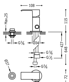
Grifo monomando para bidé con transferencia a duchita Latiguillos de alimentación flexibles G3/8.
