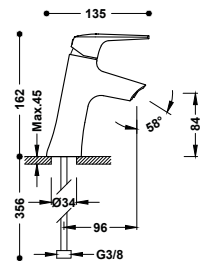
Grifo monomando inclinado para lavabo Latiguillos de alimentación flexibles G3/8.
