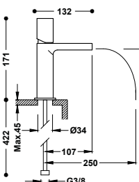
Grifo monomando para lavabo Caño abierto con salida del agua en cascada. Latiguillos de alimentación flexibles G3/8. Se incluyen 2 llaves de regulación con filtro (ref: 9134525).
