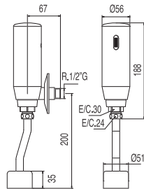
Grifo de descarga electrónico mural de 1 agua para urinario Accionado mediante sensor de infrarrojos. Con dos tubos adaptables a urinario.
