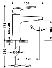
Grifo monomando ecoeficiente para lavabo Latiguillos de alimentación flexibles G3/8.
