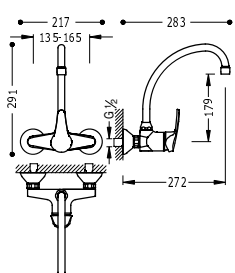
Grifo monomando mural para cocina
