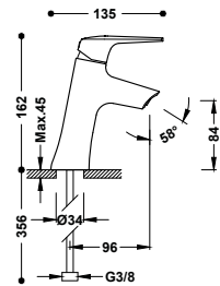
Grifo monomando inclinado ecoeficiente para lavabo Latiguillos de alimentación flexibles G3/8.
