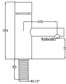
Grifo temporizado lavabo INOX
