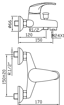
Mezclador exterior con inversor baño ducha
