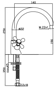
Grifo monobloque para lavabo
