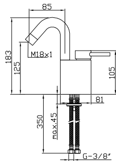
Grifo mezclador para lavabo
