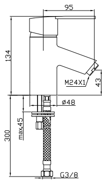
Grifo mezclador para lavabo
