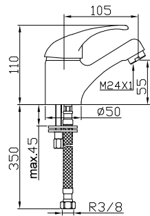
Grifo mezclador para lavabo
