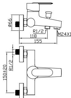
Mezclador exterior con inversor baño ducha
