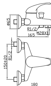
Mezclador exterior con inversor baño ducha
