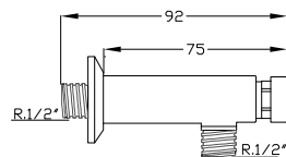
Grifo ducha de 1/2"
