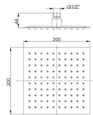
Rociador ducha cuadrado INOX
