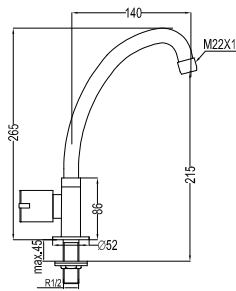
Grifo fregadero caño vertical/ giratorio
