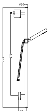
Kit de ducha PRISMA c/ mango de ducha
