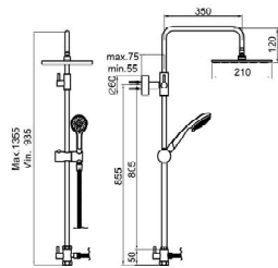
Barra de ducha vista telescópica para grifería baño ducha
