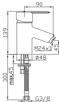
Grifo mezclador para lavabo
