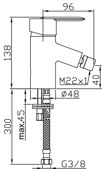
Grifo mezclador para bidé
