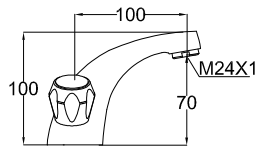
Grifo monobloque para lavabo Mono basin mixer Mélangeur lavabo
