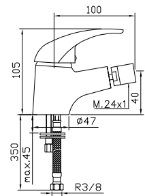
Grifo mezclador para bidé
