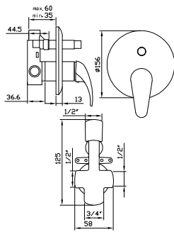
Monomando baño ducha empotrado Concealed bath-shower Mitigeur bain douche à encastrer
