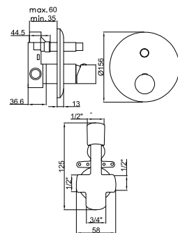
Monomando ducha empotrado con dos salidas Concealed bath-shower with two outputs Mitigeur douche a encastrer avec deux sorties
