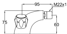
Grifo monobloque para bidé con rótula Mono bidet mixer Mélangeur bidet
