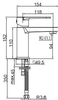
Grifo mezclador para lavabo alto
