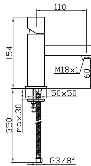
Monomando de lavabo Basin mixer Mitigeur lavabo
