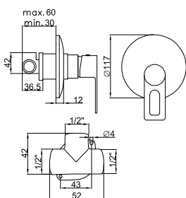
Monomando ducha empotrado Concealed shower Mitigeur douche a encastrer
