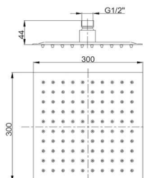
Rociador ducha cuadrado INOX
