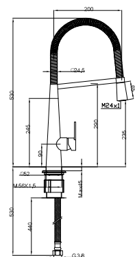
Grifo mezclador para fregadero con muelle extensible
