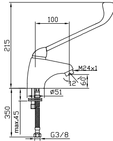
Grifo mezclador para lavabo con palanca gerontológica
