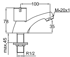
Grifo de repisa para lavabo con aireador
