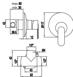
Monomando ducha empotrado
