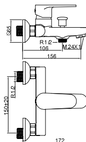
Mezclador exterior con inversor baño ducha
