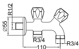
Grifo para lavadora doble 3/4" Double mixer for washing machine 3/4" Robinet double pour machine à laver 3/4"
