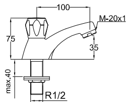
Grifo de repisa para lavabo con atomizador Basin tap Robinet simple pour lavabo
