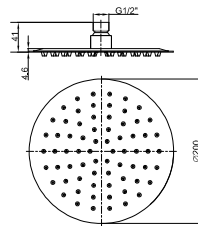
Rociador ducha INOX
