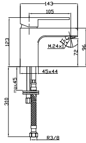
Monomando lavabo Basin mixer Mitigeur lavabo
