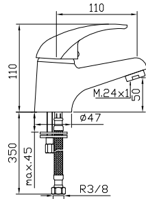
Grifo mezclador para lavabo
