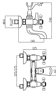
Mezclador exterior con inversor baño-ducha
