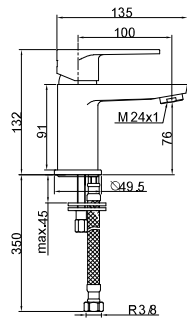
Grifo mezclador para lavabo
