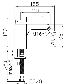
Monomando de bidé Bidet mixer Mitigeur bidet
