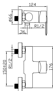
Mezclador exterior para ducha
