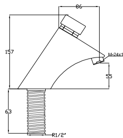
Grifo temporizado de lavabo en latón cromado
