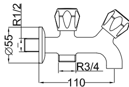
Grifo para lavadora doble Double mixer for washing machine Robinet double pour machine à laver
