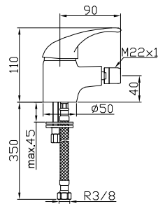
Grifo mezclador para bidé
