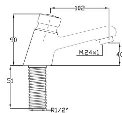
Grifo temporizado de lavabo en latón cromado
