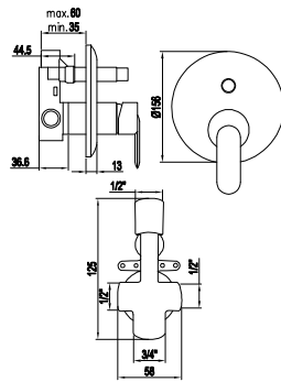
Monomando baño ducha empotrado
