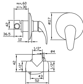
Monomando ducha empotrado Concealed shower Mitigeur douche a encastrer
