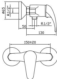
Mezclador exterior para ducha
