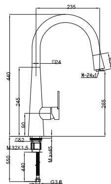
Grifo mezclador para fregadero con ducha extraíble
