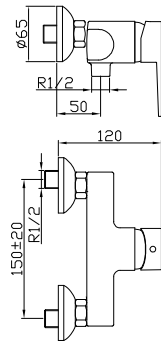
Mezclador exterior para ducha
