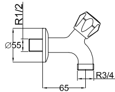
Grifo de lavadora 1/2", salida 3/4" Mixer for washing machine, 1/2"-3/4" Robinet pour machine à laver 1/2"-3/4"
