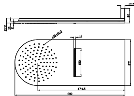
Rociador con cascada slim inox
