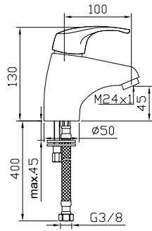
Grifo mezclador para lavabo
