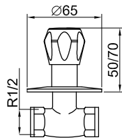
Llave de paso para empotrar 1/2 "G Remote control valve, 1/2" Robinet d'arrêt 1/2 " encastré
