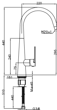
Grifo mezclador para fregadero
