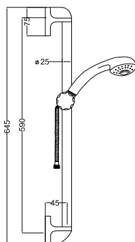
Kit de ducha LUNA c/ mango 3 posiciones orientable
