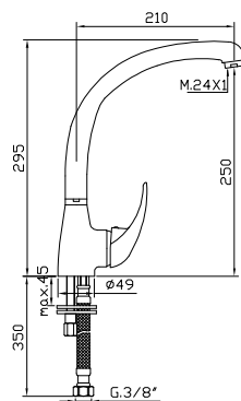
Grifo mezclador para fregadero de repisa caño de tubo conformado Sink mixer with formed spout Mitigeur évier bec mobile haut tube
